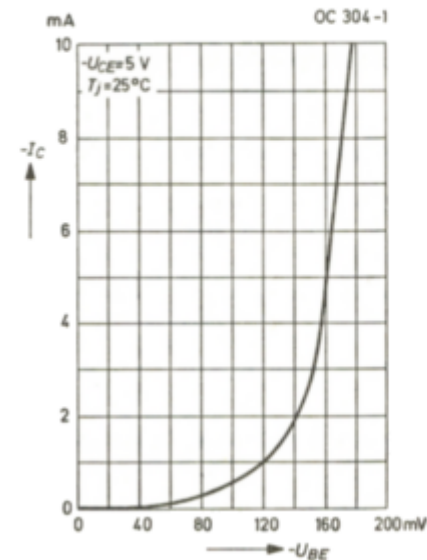
Steilheit des OC 304-1 -I_C = f(-U_{BE})
