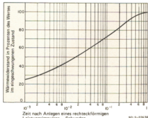
Bild 12: Einschwing-Wärmewiderstand zwischen Sperrschicht und Gehäuse in Abhängigkeit von der Zeit für alle Typen
