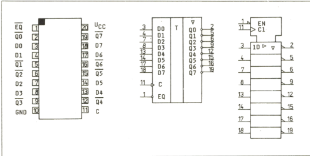
Anschlußbelegung, Schaltzeichen und IEC-Zeichen
